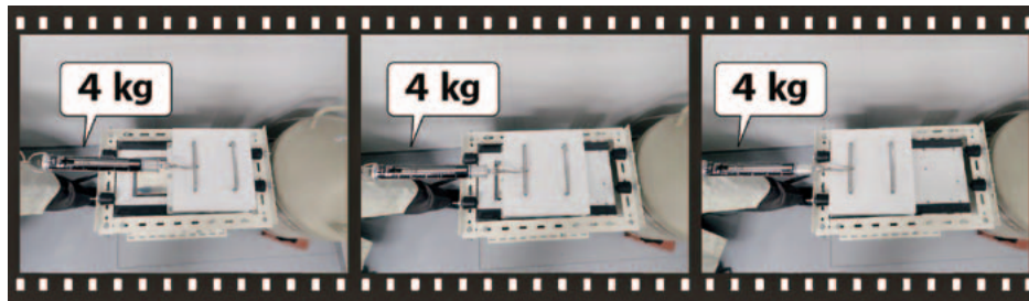
図6 スベリ機構による鉛遮蔽蓋の開閉に必要な力の測定（オイレスシートに潤滑油を塗布した場合）
