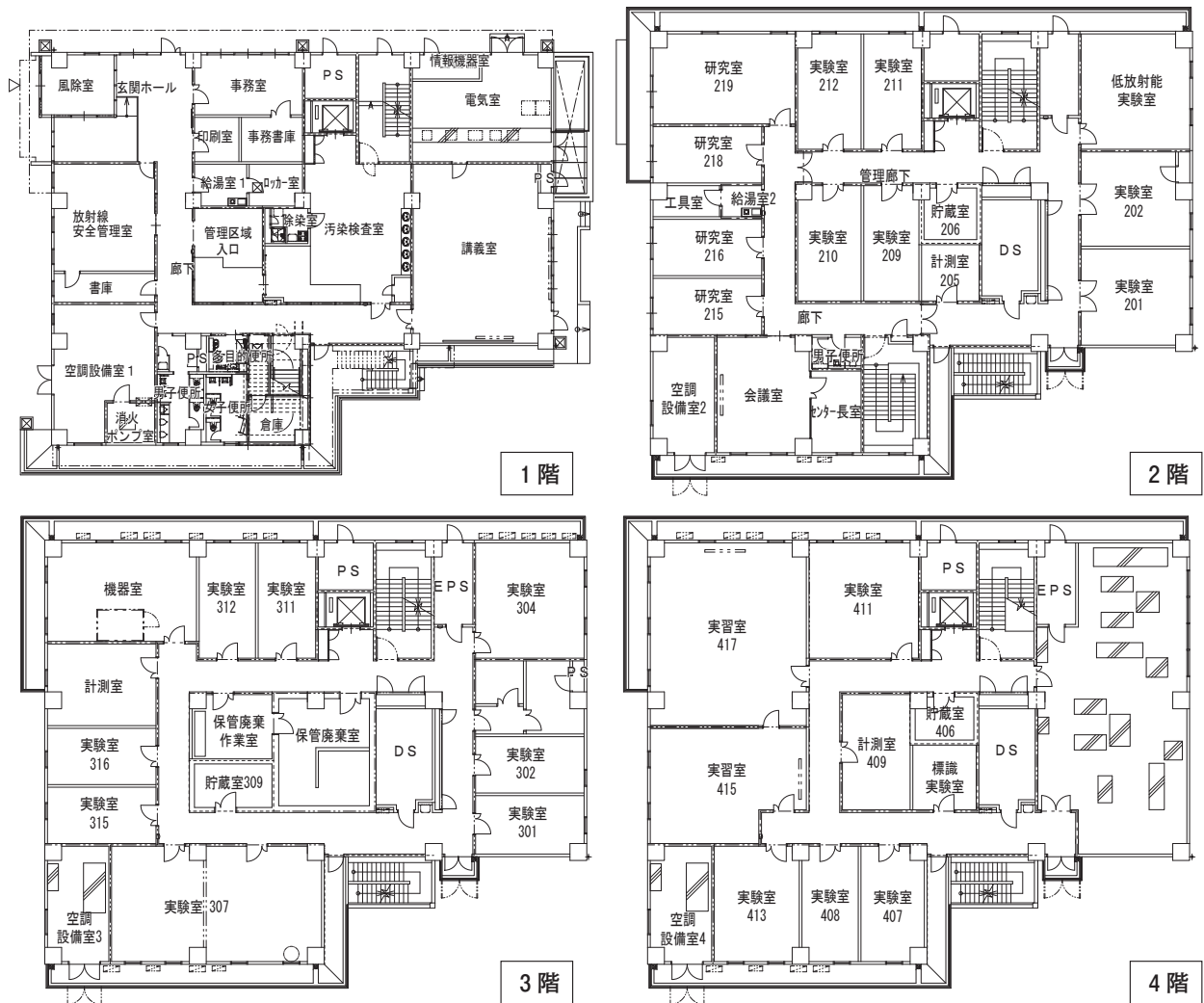
図1 新RI実験棟平面図（1階～4階）
