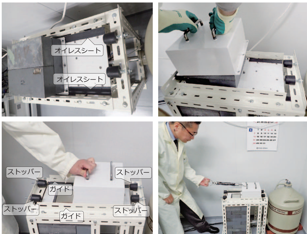
図2 スベリ機構による鉛遮蔽蓋の開閉
